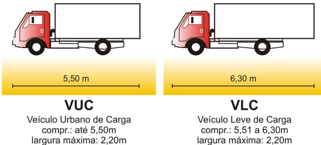
Figura 4 – Dimensões antigas do Veículo Urbano de Carga e do Veículo Leve de Carga – Decreto 37.185/97
